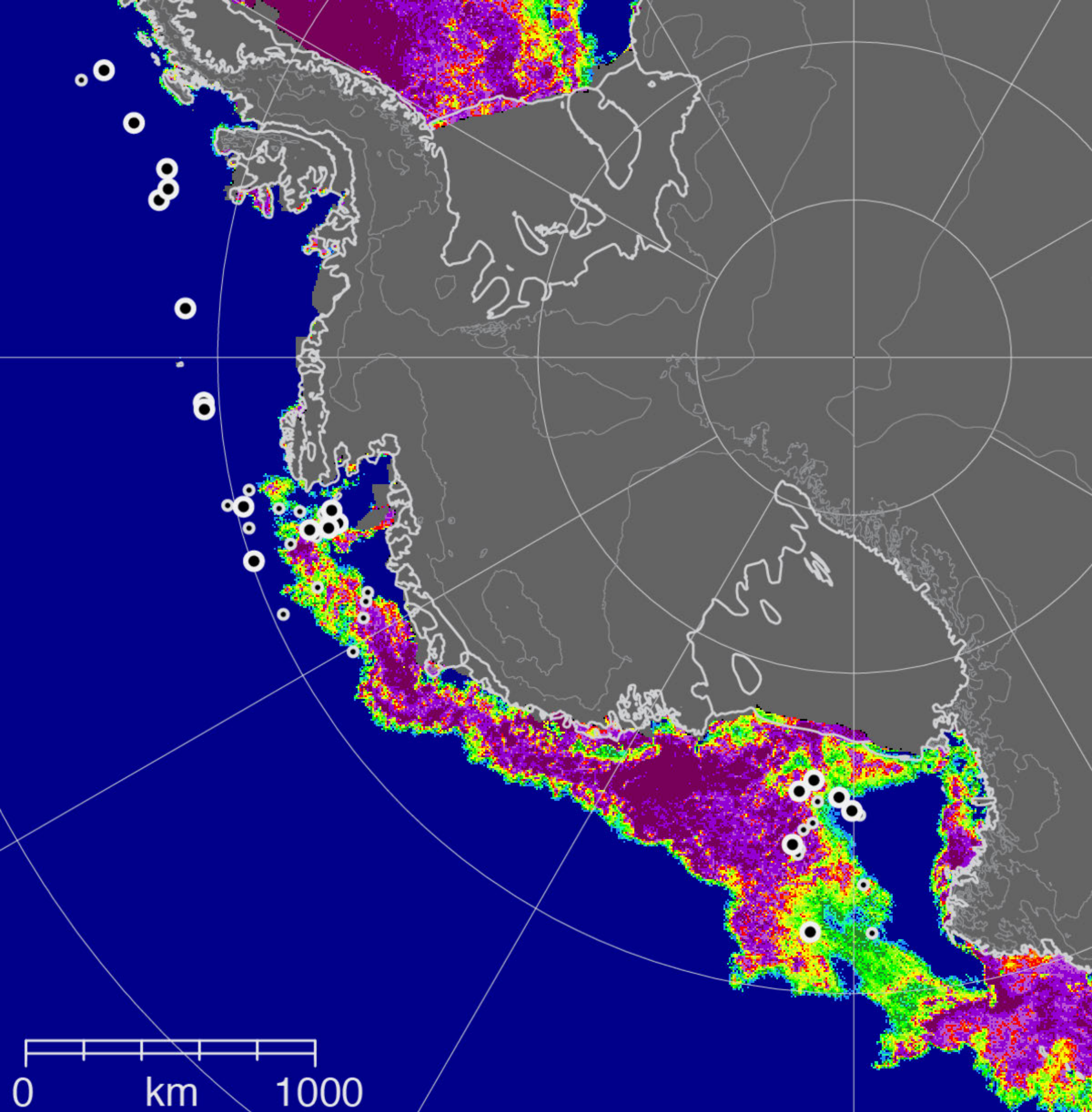
AMSR2 sea ice: 2013-03-04
