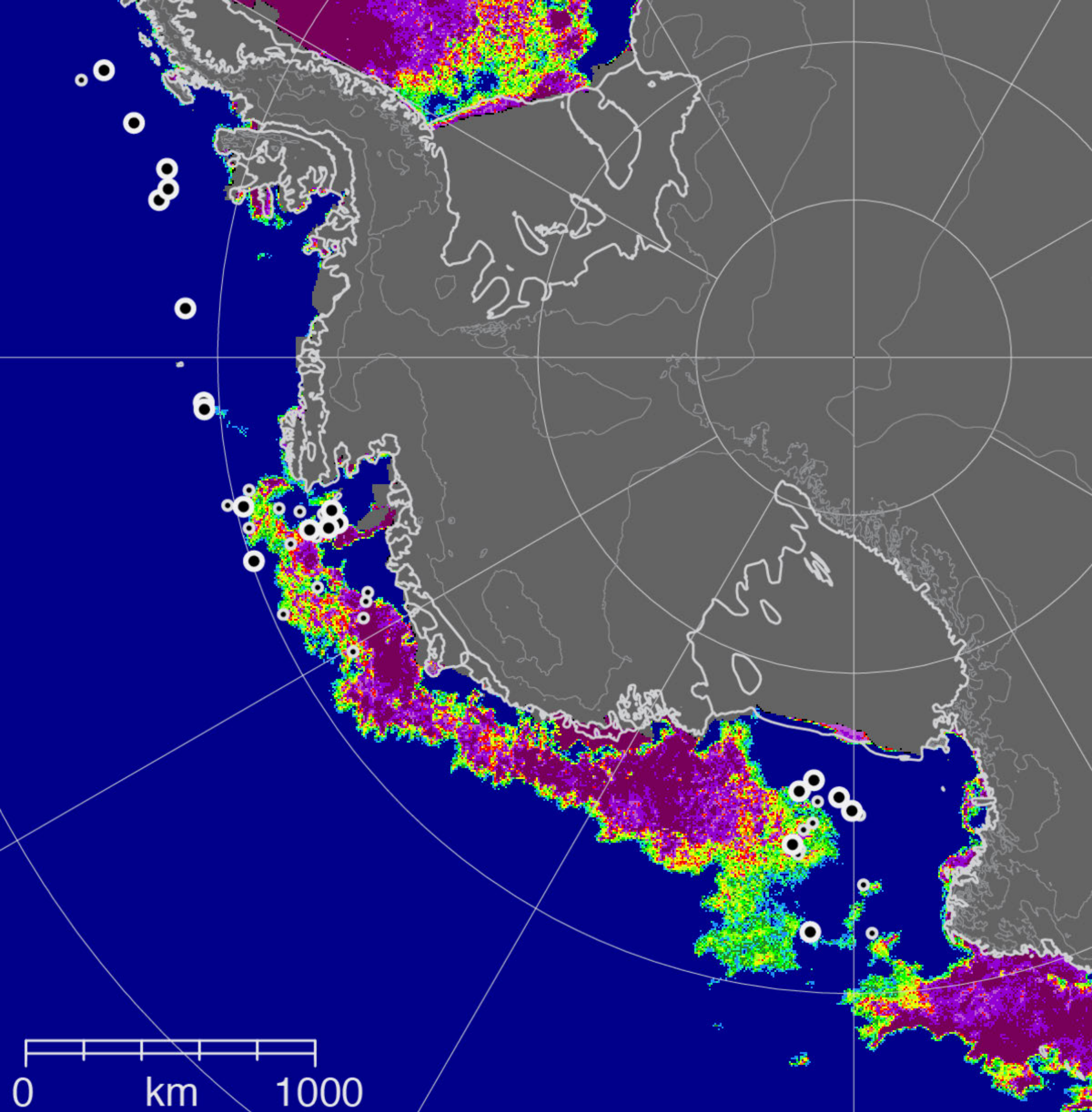
AMSR2 sea ice: 2013-02-11
